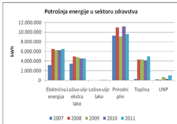
Slika 10 Potrošnja energije u sektoru zdravstva
