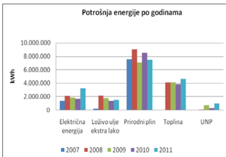
Slika 6 Prikaz ukupne potrošnje energije po godinama u kWh
