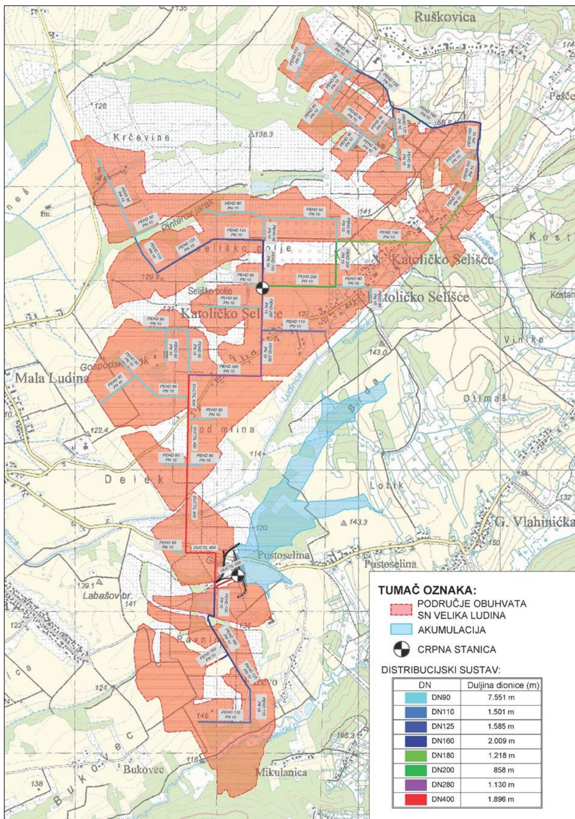
Slika 2. Pregledna situacija odabranog optimalnog varijantnog rješenja SN Velika Ludina (Izvor: Novelacija studije Izvodljivosti, listopad 2022. g.)
