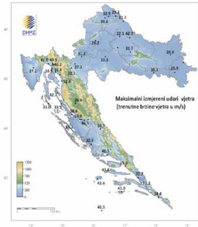
Slika 1: Maksimalni izmjereni udari vjetra (trenutne brzine vjetra) na meteorološkim postajama u Hrvatskoj Izvor podataka: Izmjene i dopune studije meteorološka podloga za potrebe procjene ugroženosti RH od prirodnih i tehničko-ehnoloških katastrofa i velikih nesreća, prosinac 2011. godine
