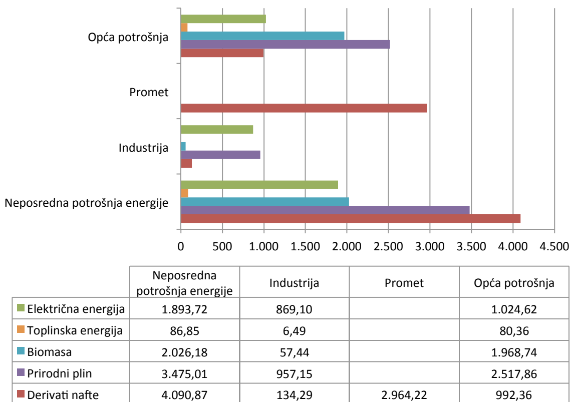
Slika 34: Dijagram toka energije u neposrednoj potrošnji [TJ]
