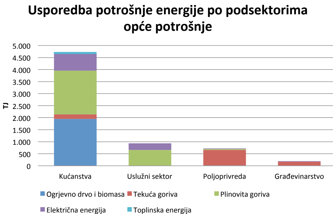
Slika 26: Usporedba potrošnje energije po podsektorima opće potrošnje
